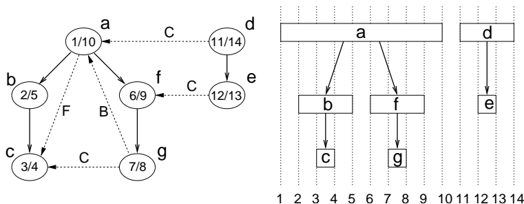
Fig. 26: Parenthesis Lemma.
