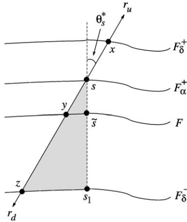
Fig. 14. Illustration for Lemma 8.4.
