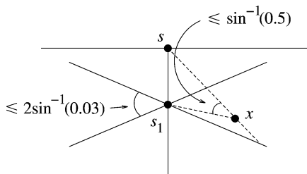
Fig. A.3. Illustration for Lemma 7.4.
