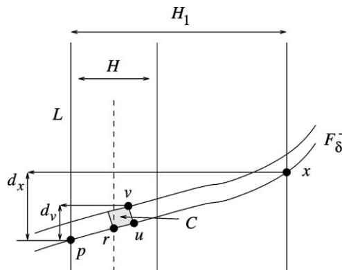
Fig. 12. Illustration for Lemma 8.3.
