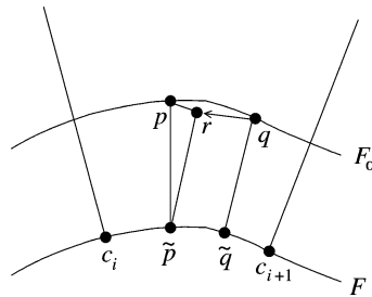
Fig. 7. Illustration for Lemma 6.1.
