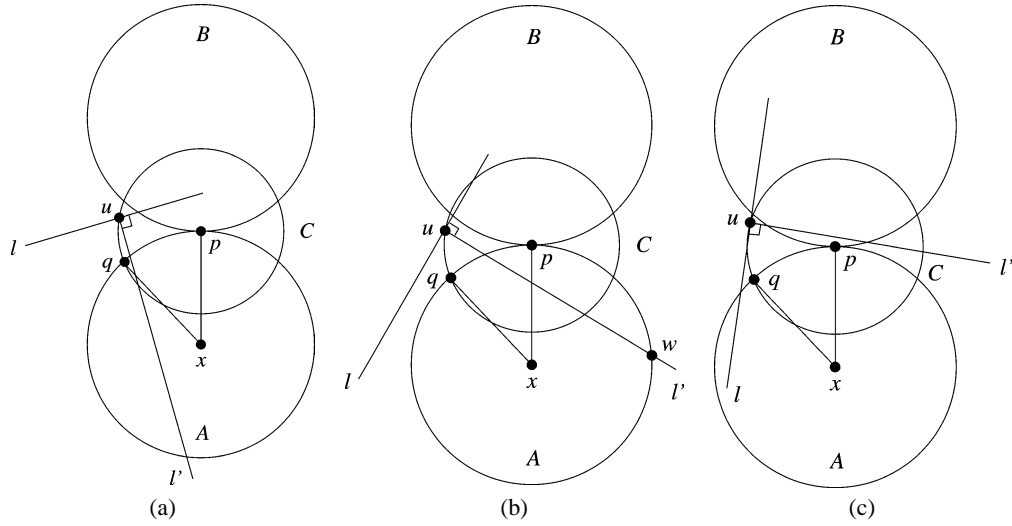
Fig. A.2. Illustration for Lemma 5.3.
