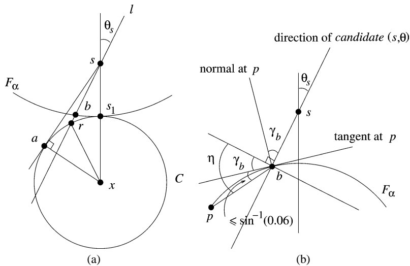
Fig. A.5. Illustration for Lemma 8.1(iv).
