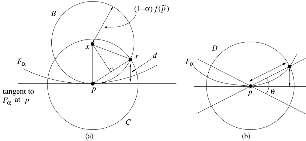
Fig. A.1. Illustration for Lemma 5.2.
