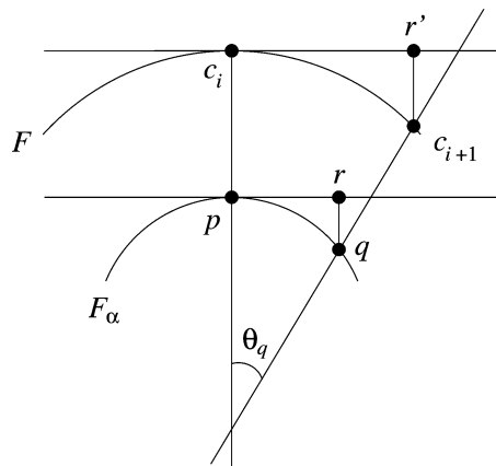
Fig. 8. Illustration for Lemma 6.3.
